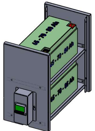
NC00 - 65-70-80Ah x 2
