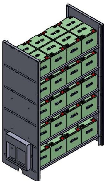
NC51 - 40Ah x 40
