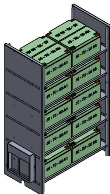
NC51 - 65-70-80Ah x 20
