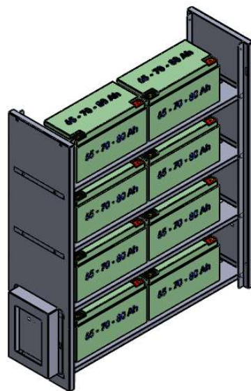
NC30 - 65-70-80Ah x 8
